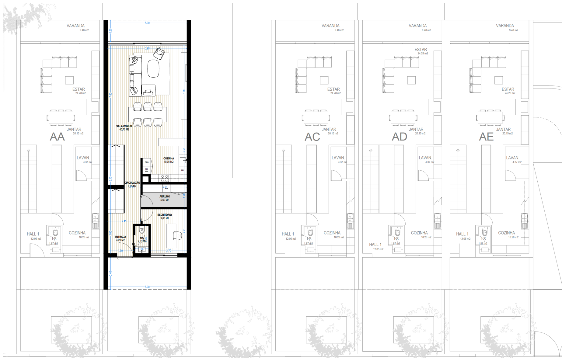
PLANTA PISO 0
