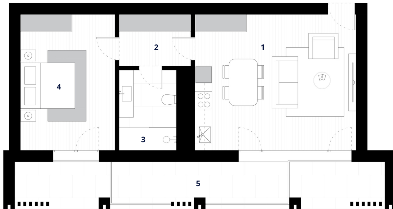
PISO 4
