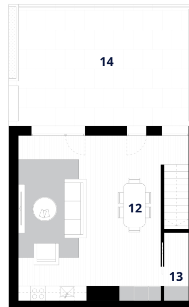
PISO -1
