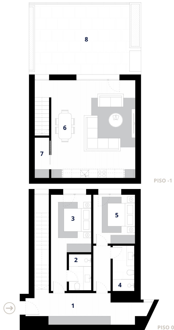
PISO 0
