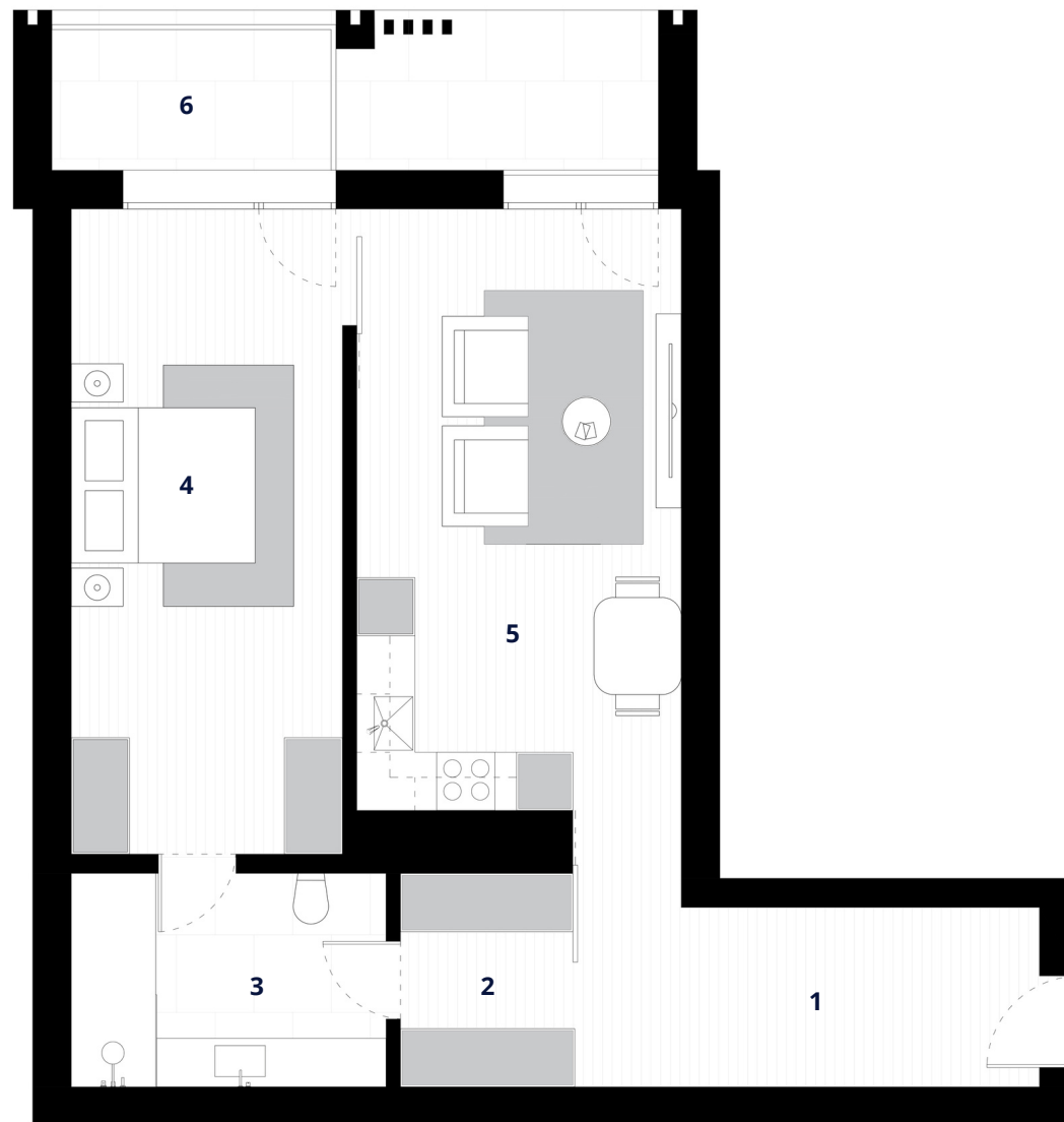
PISO 2
