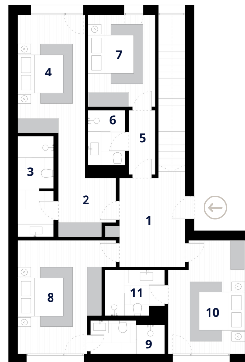
PISO -1
