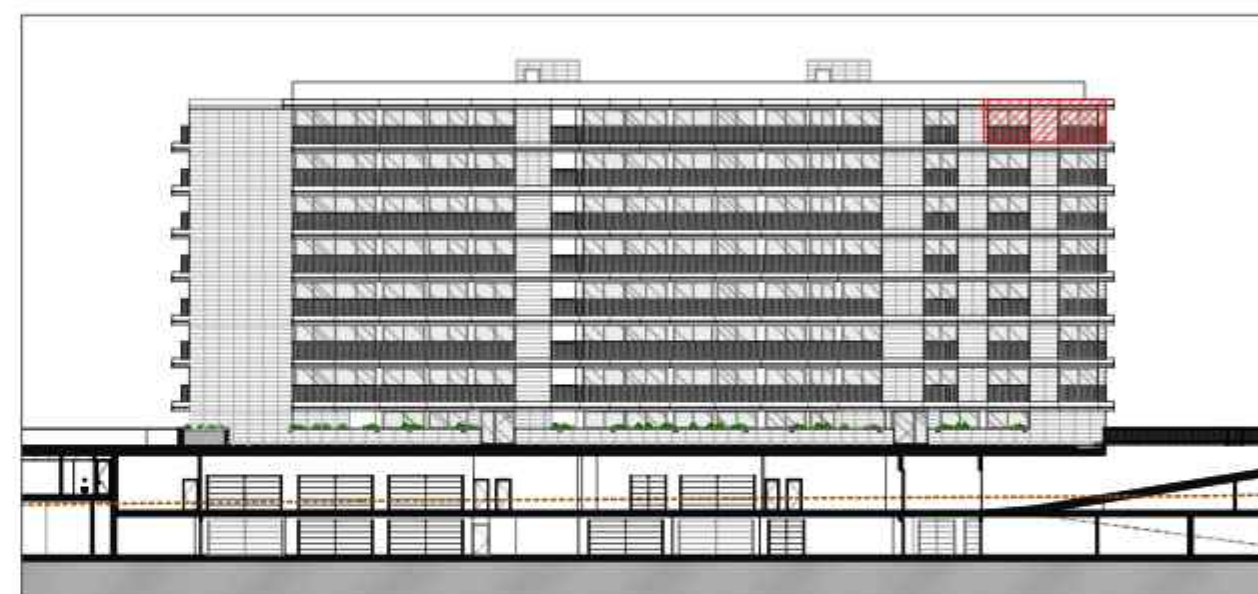
ALÇADO NASCENTE 1/500
