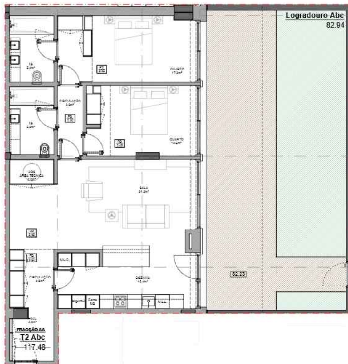
PLANTA 1/100
