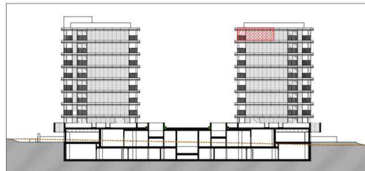
ALÇADO NORTE 1/500
