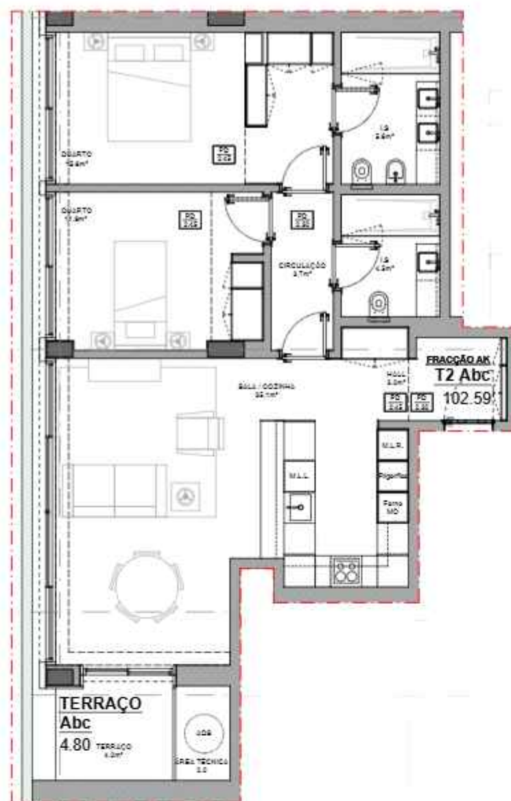
PLANTA 1/100
