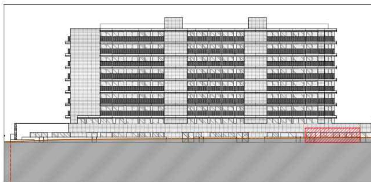
ALÇADO NASCENTE 1/500
