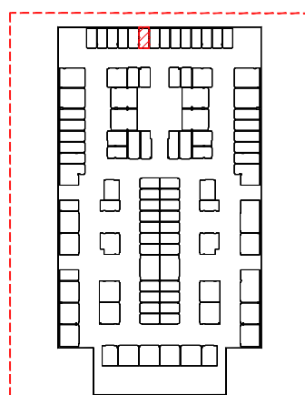
PLANTA ENQUADRAMENTO DO PISO -2
