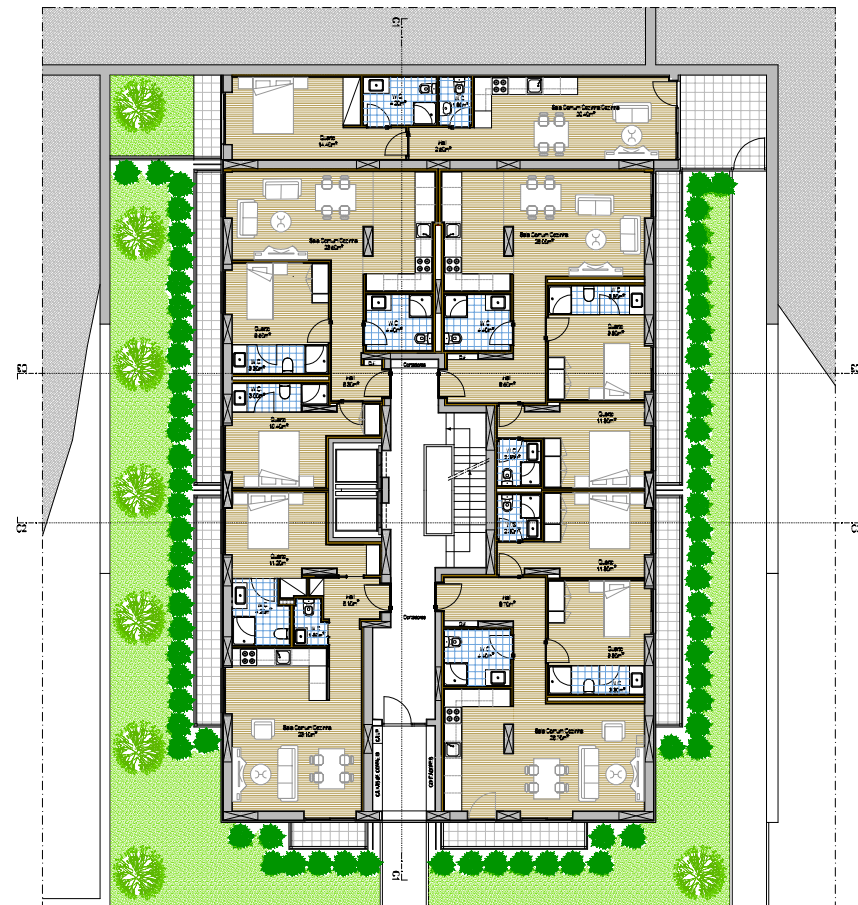
PLANTA DO PISO 1 (Cota: 0.00)
