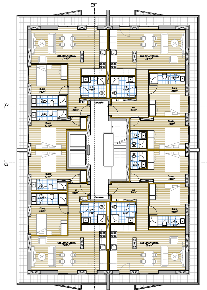
PLANTA DO PISO 9 (Cota: 23.68)
