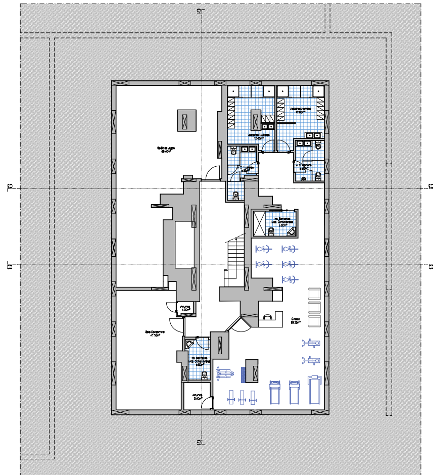
PLANTA DO PISO -1 (Cota: -2,96)
