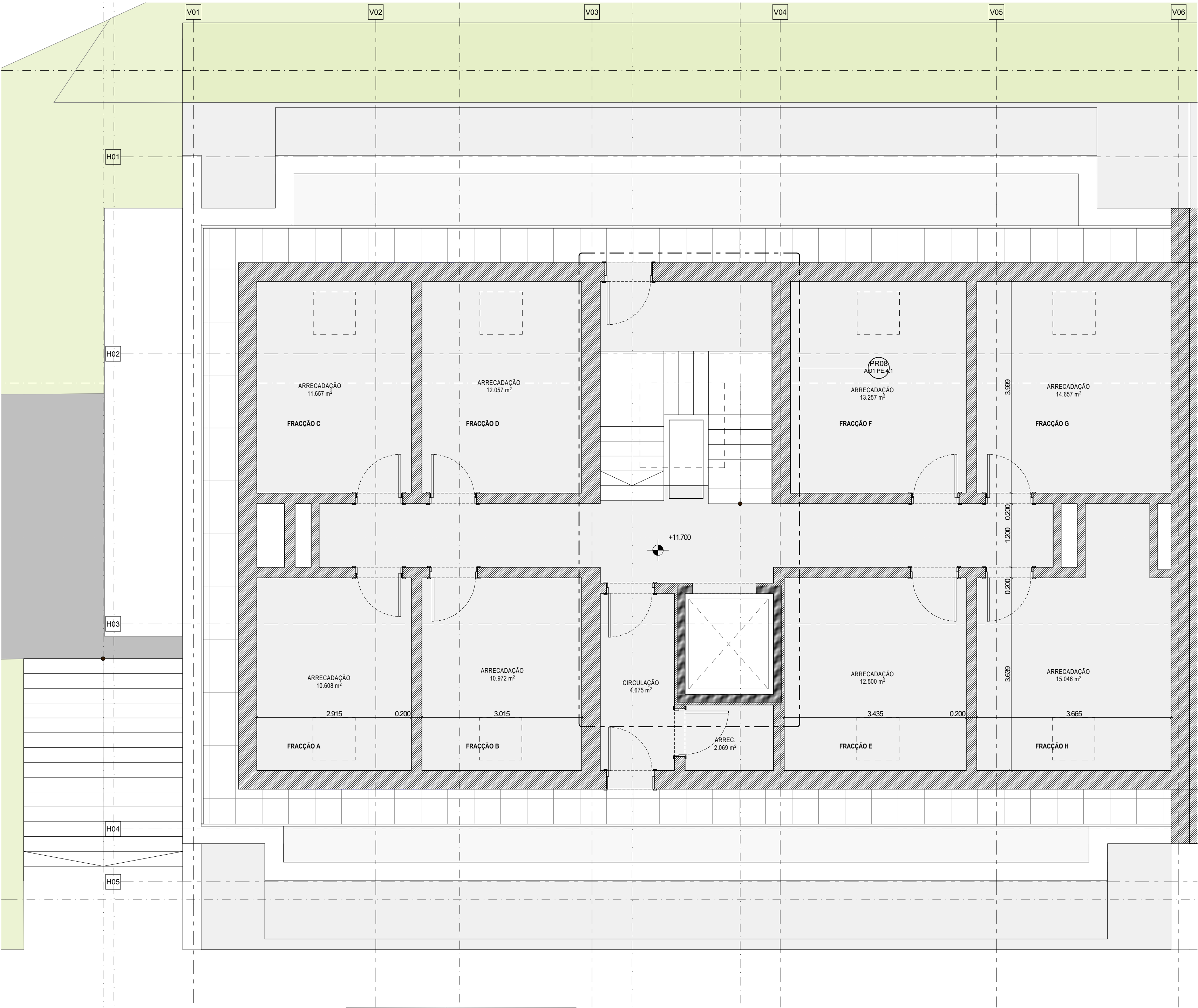
PLANTA DA COBERTURA N1
