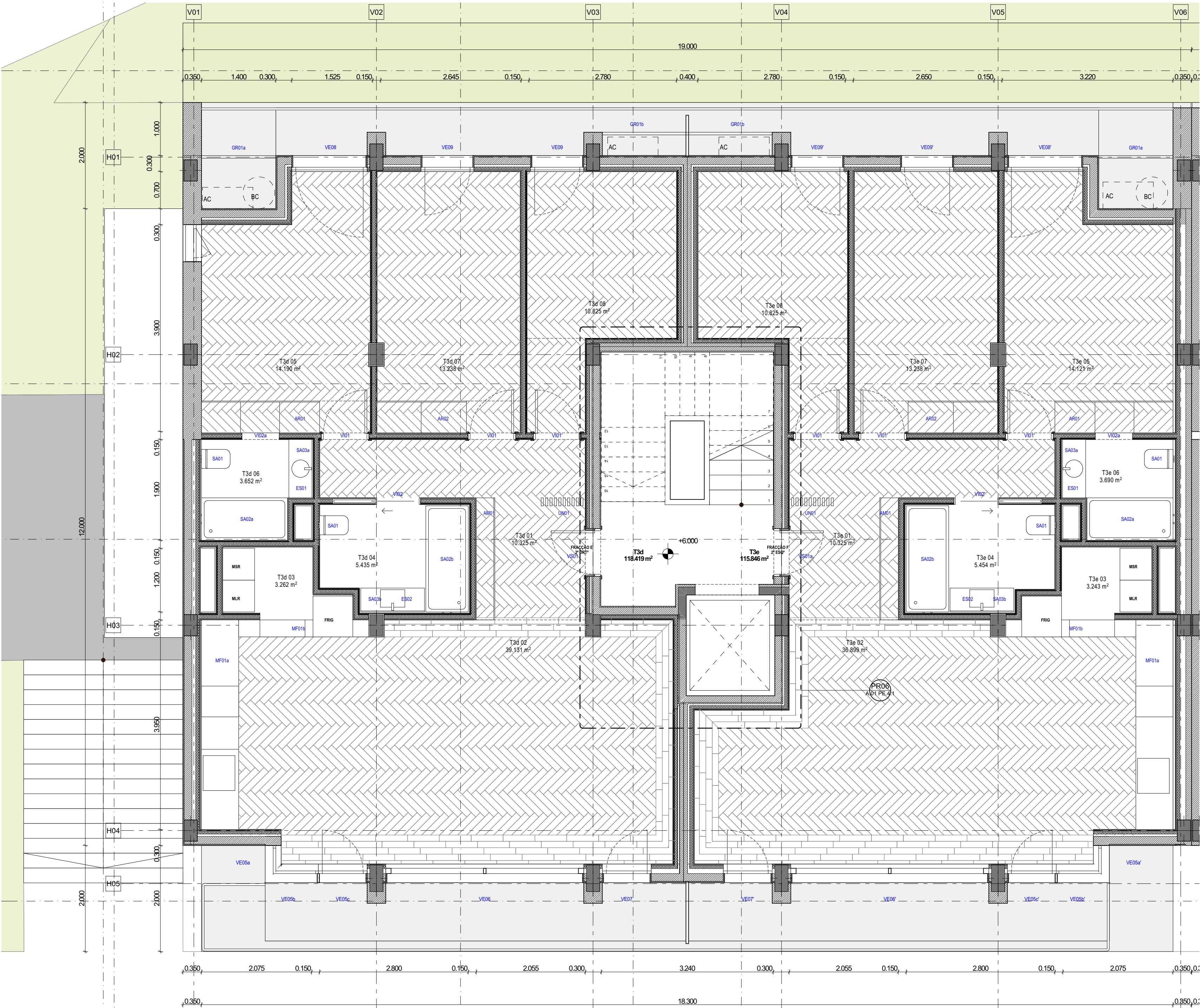
PLANTA DO PISO 2
