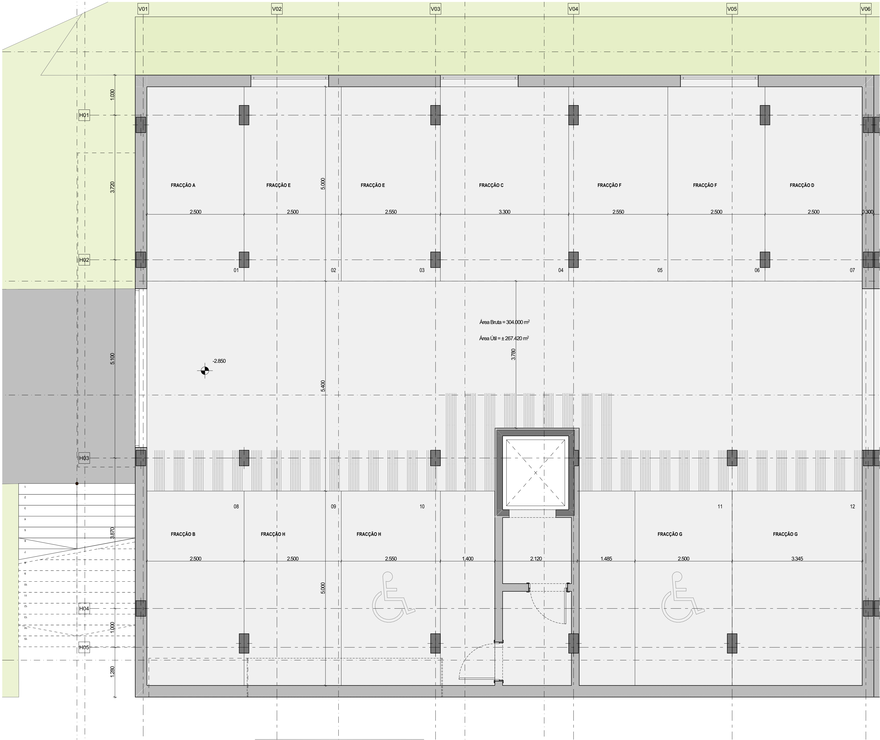
PLANTA DO PISO -1
