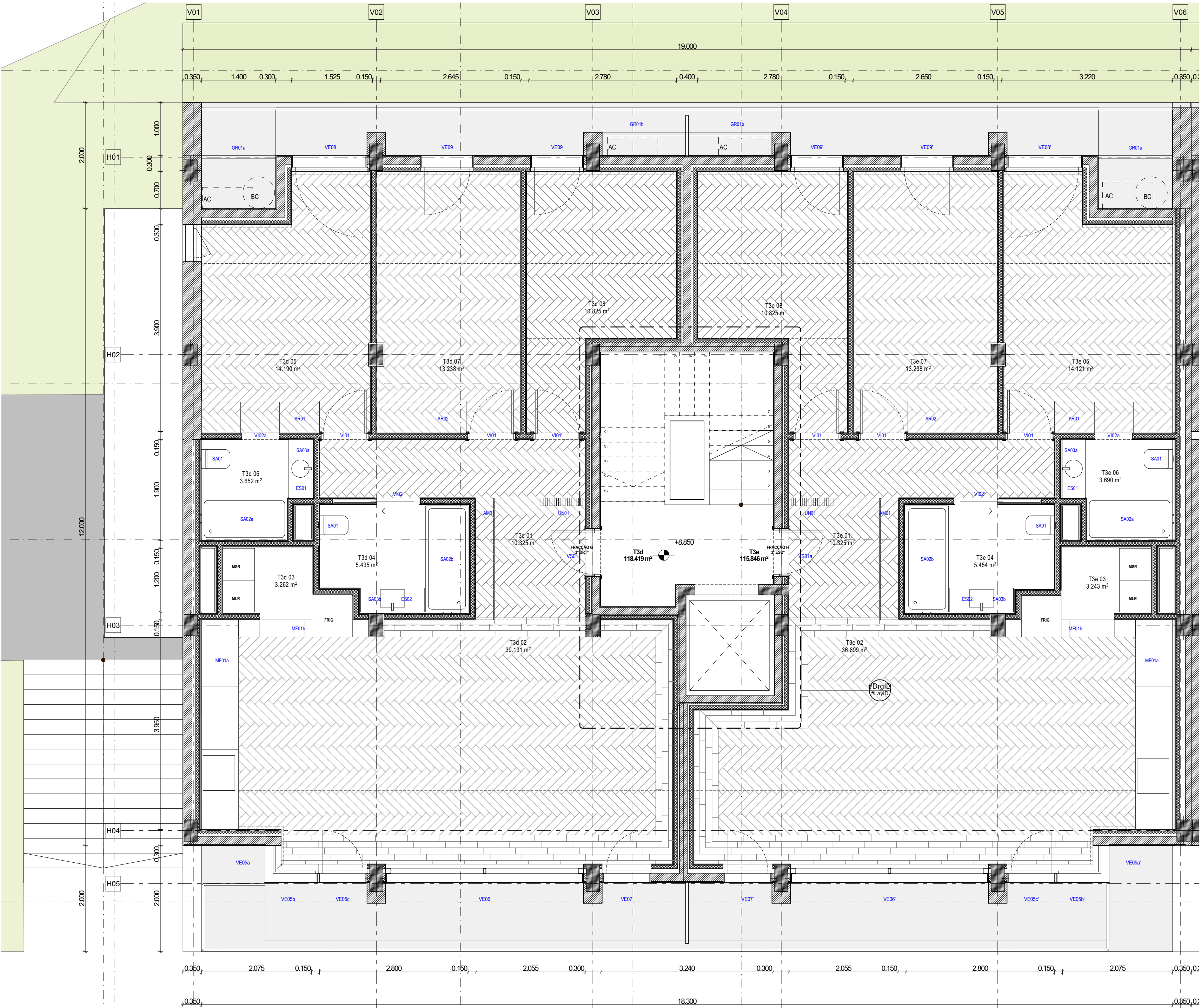
PLANTA DO PISO 3
