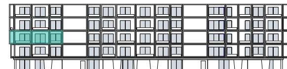
ALÇADO SUL SOUTH ELEVATION
