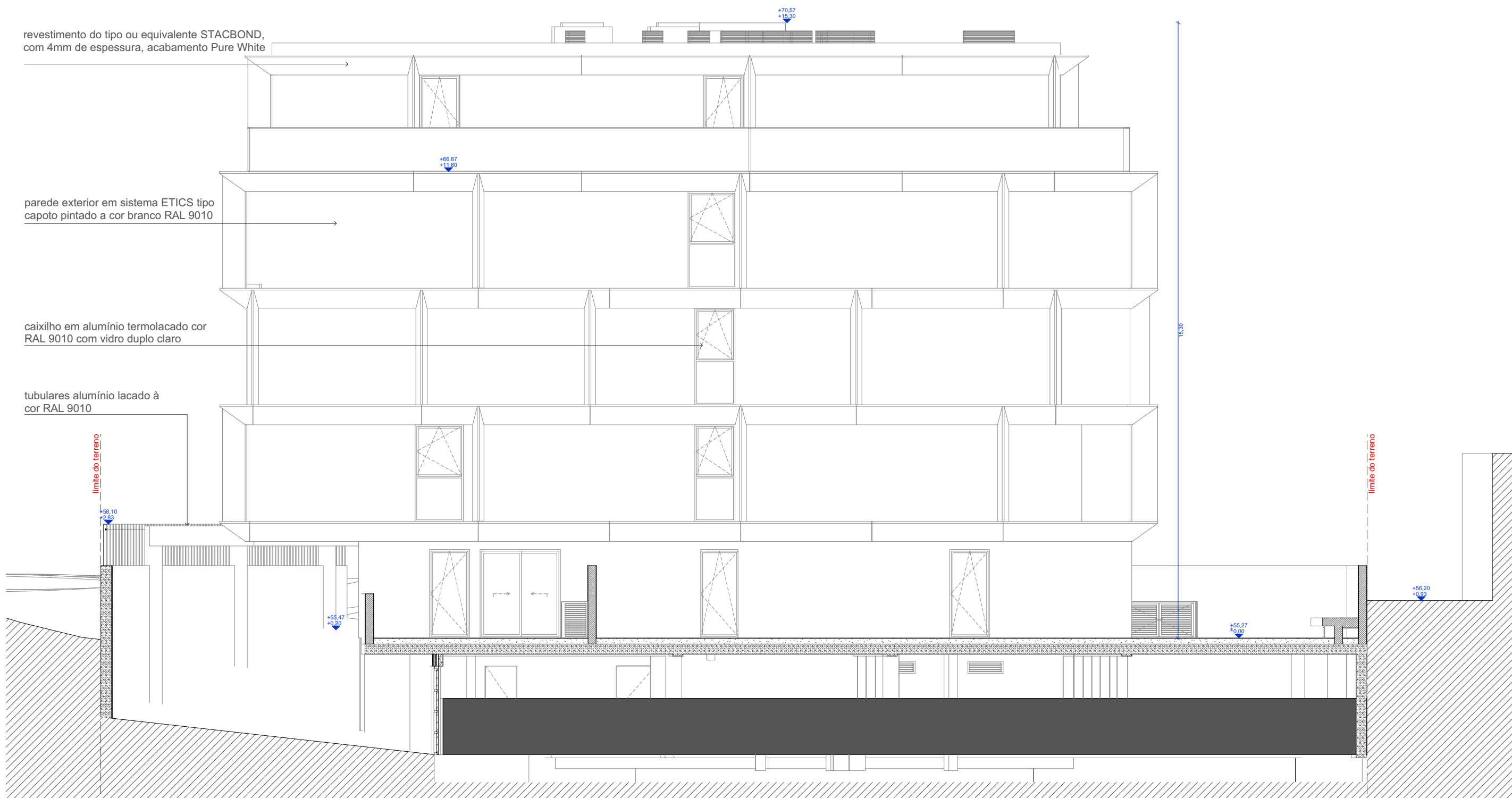
Alçado A02 - norte
