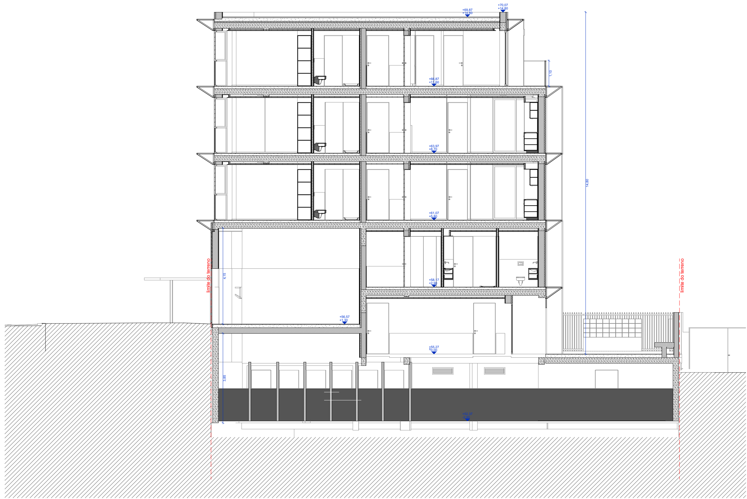
Corte C01
