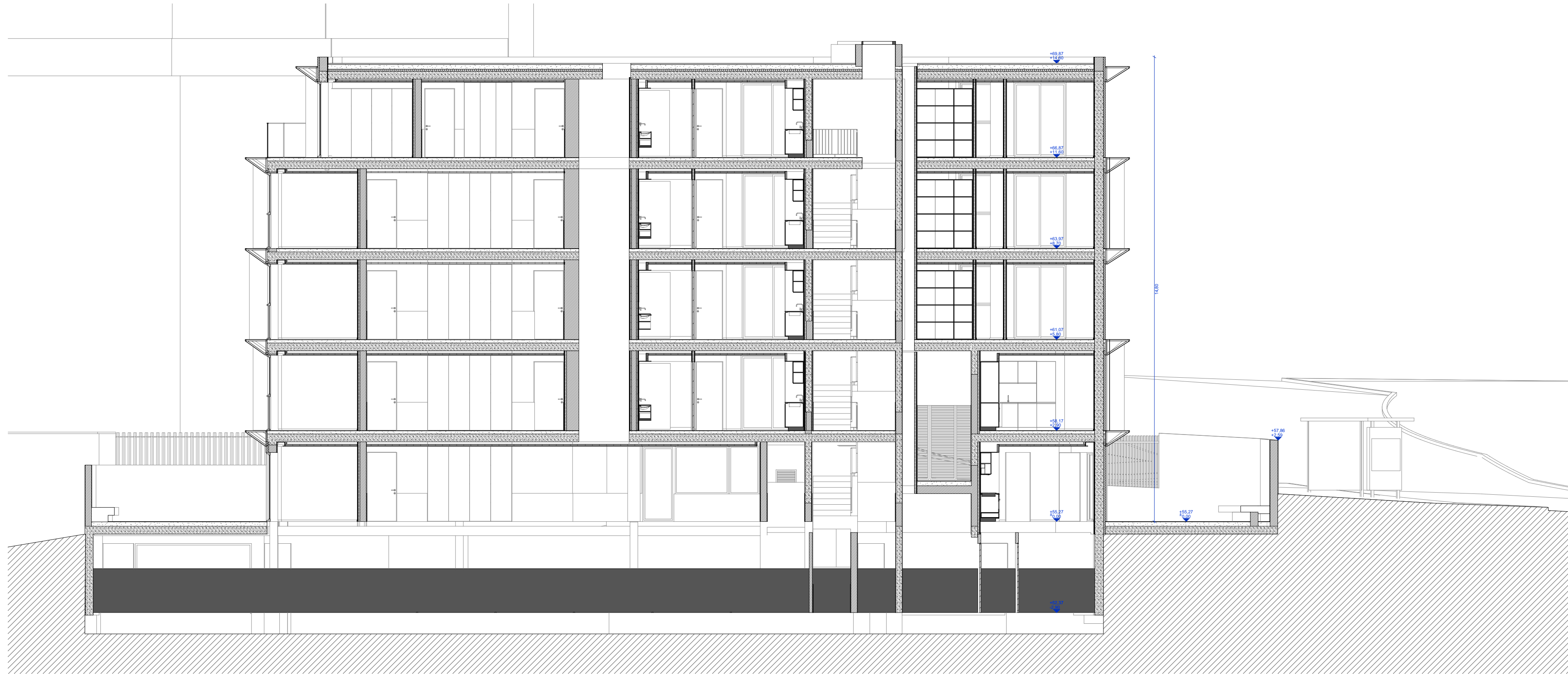
Corte C04
