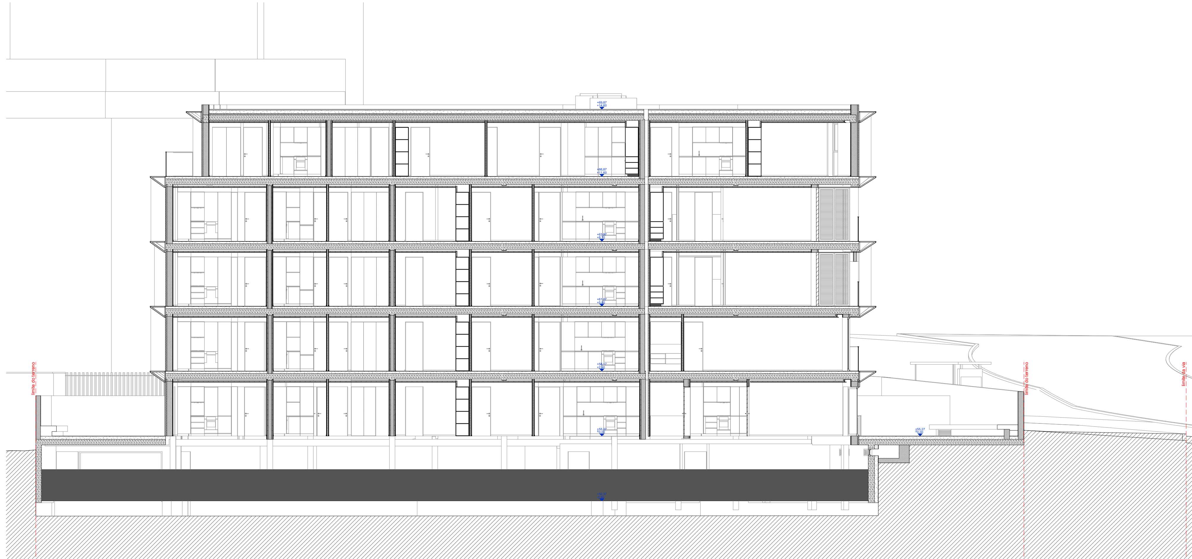
Corte C02
