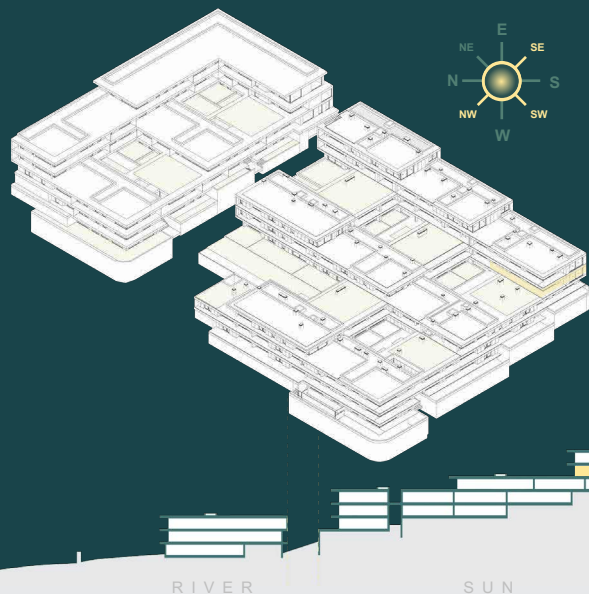
VISTA DA SECÇÃO Norte-Oeste SECTION VIEW North-West
