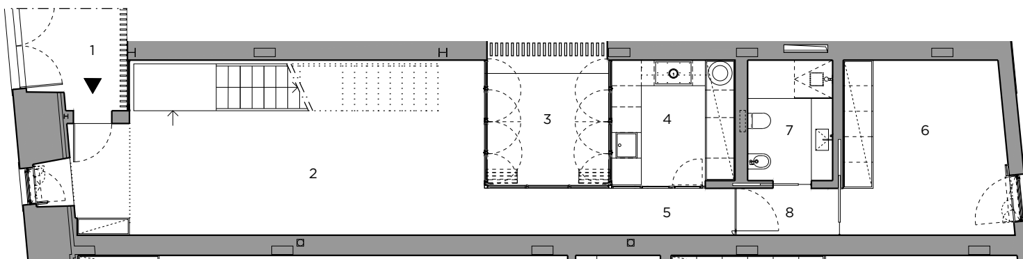
PISO 0
