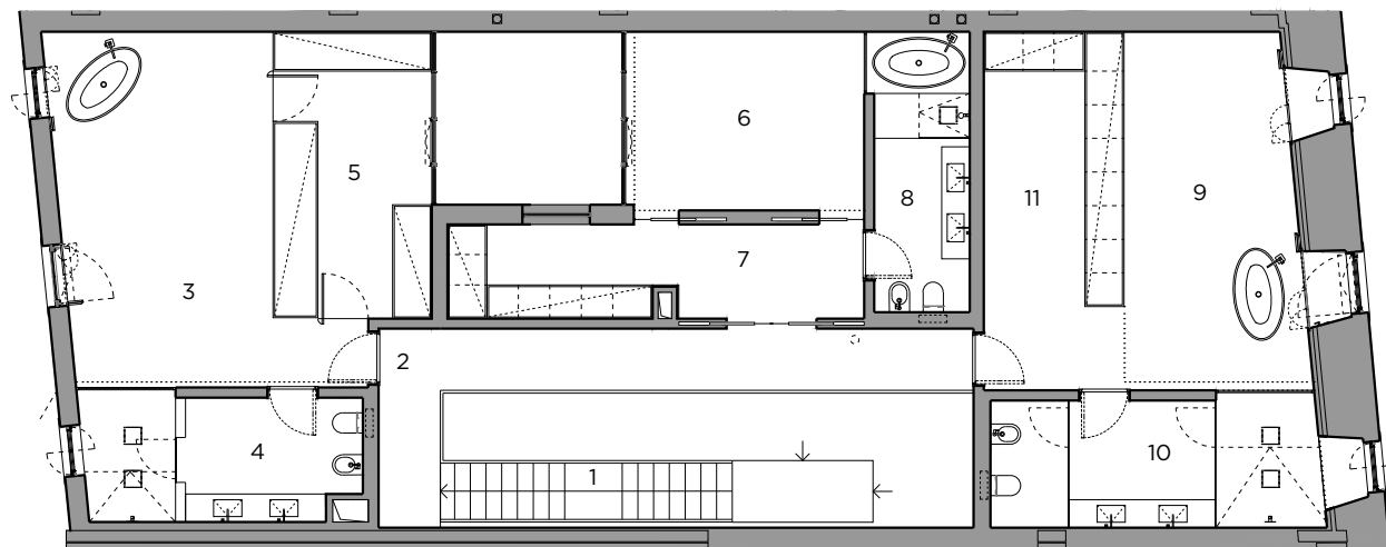
PISO 1
