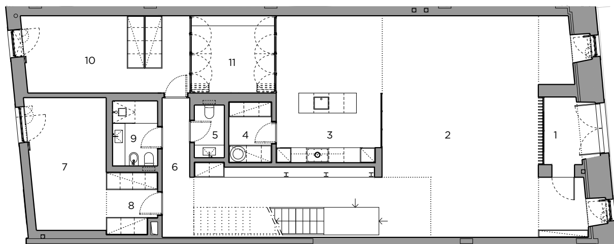
PISO 0
