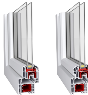
Caxilharia em pvc CAIXIAVE Serie 70 ou equivalente, na cor branco puro, com vidros duplos
