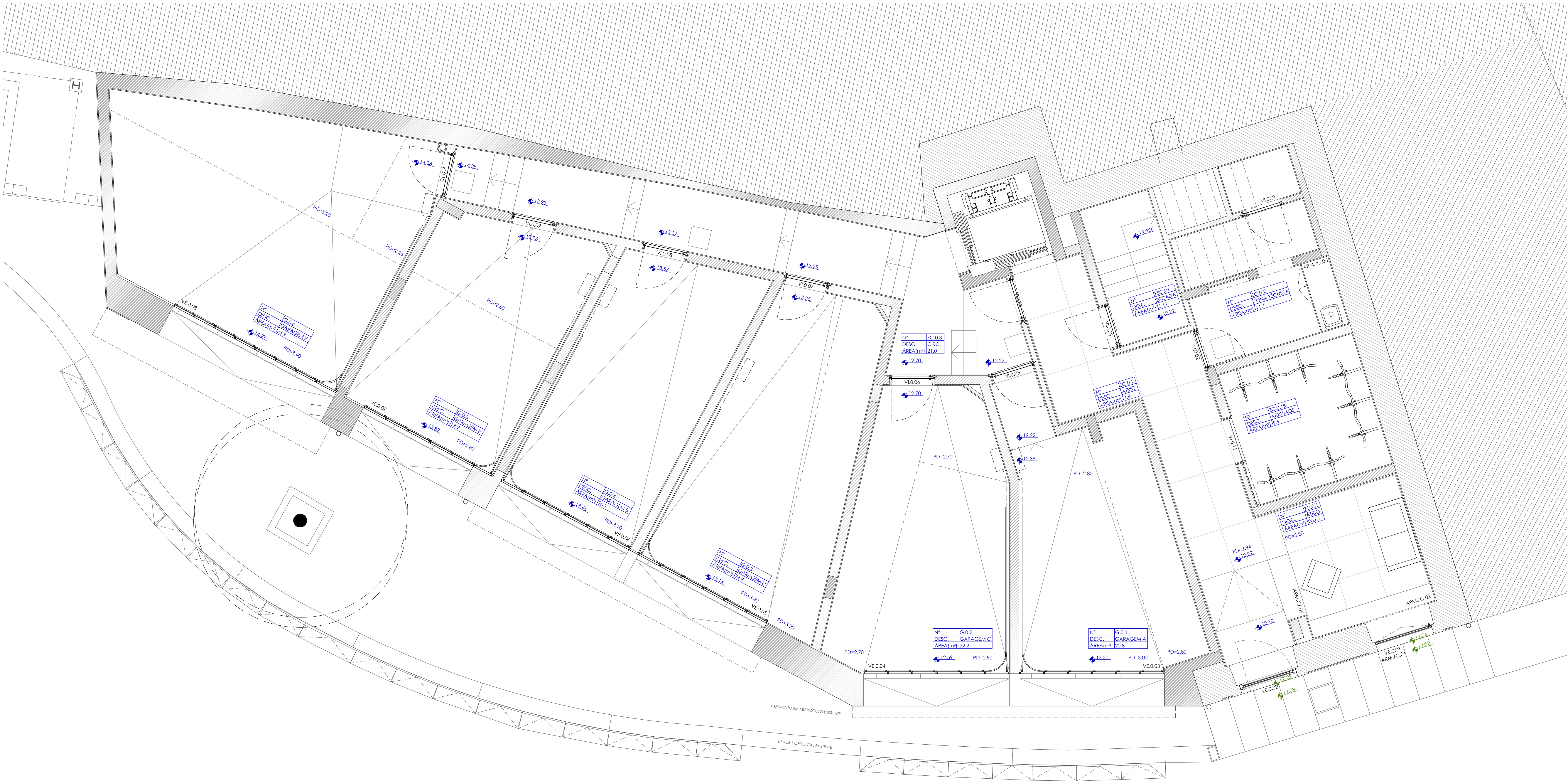
PLANTA PISO 0
