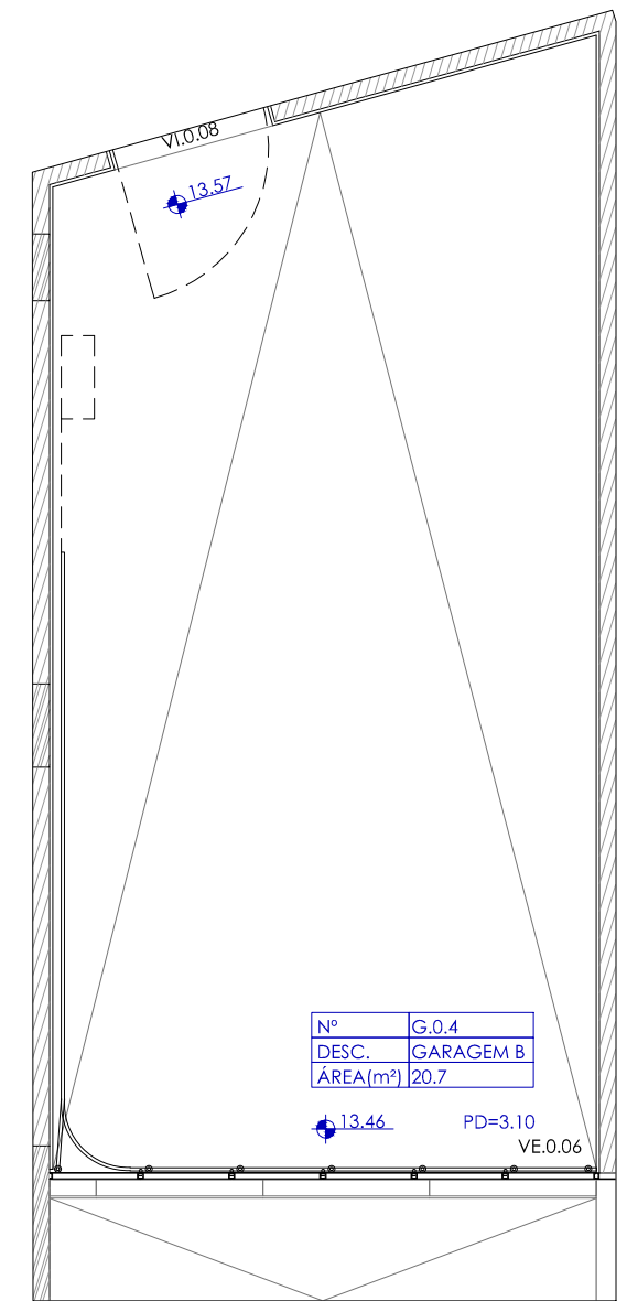
PLANTA GARAGEM FRACÇÃO B A.B.C. 25,41 m²
