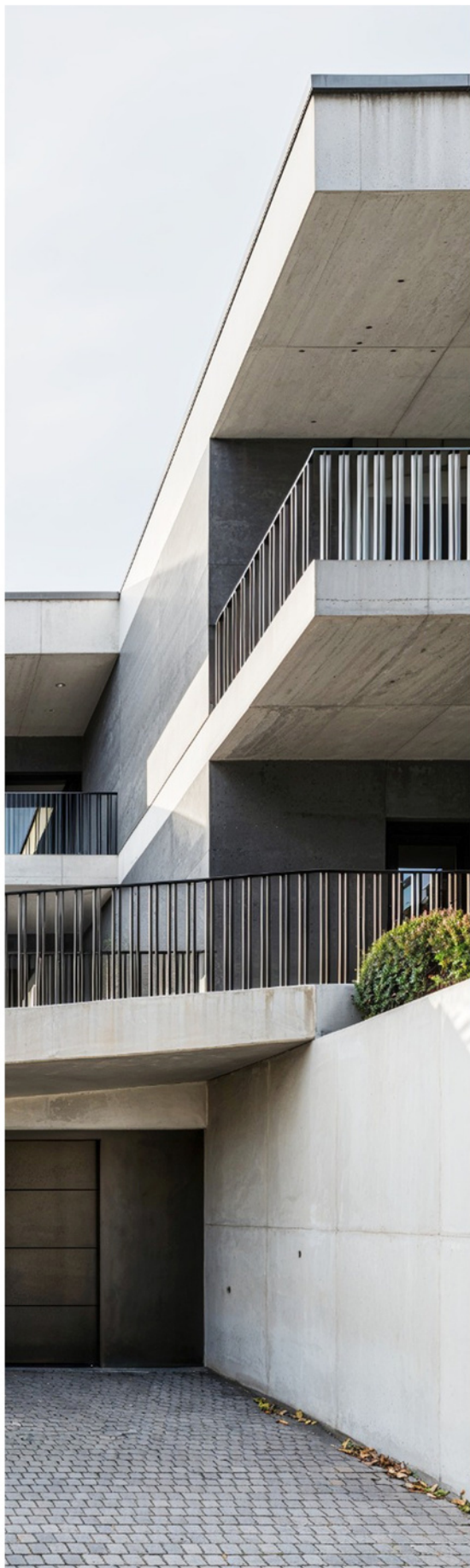
Caixilharias, Série de Correr com acabamento a RAL 7016 Mate, com vidro térmico Guardian Sun incolor
