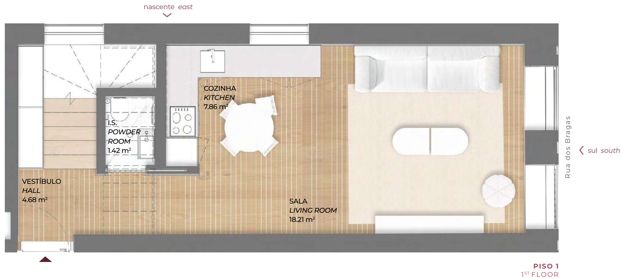
T1 / One-bedroom flat Planta de Tipologia / Typology Floorplan FRAÇÃO UNIT AB
