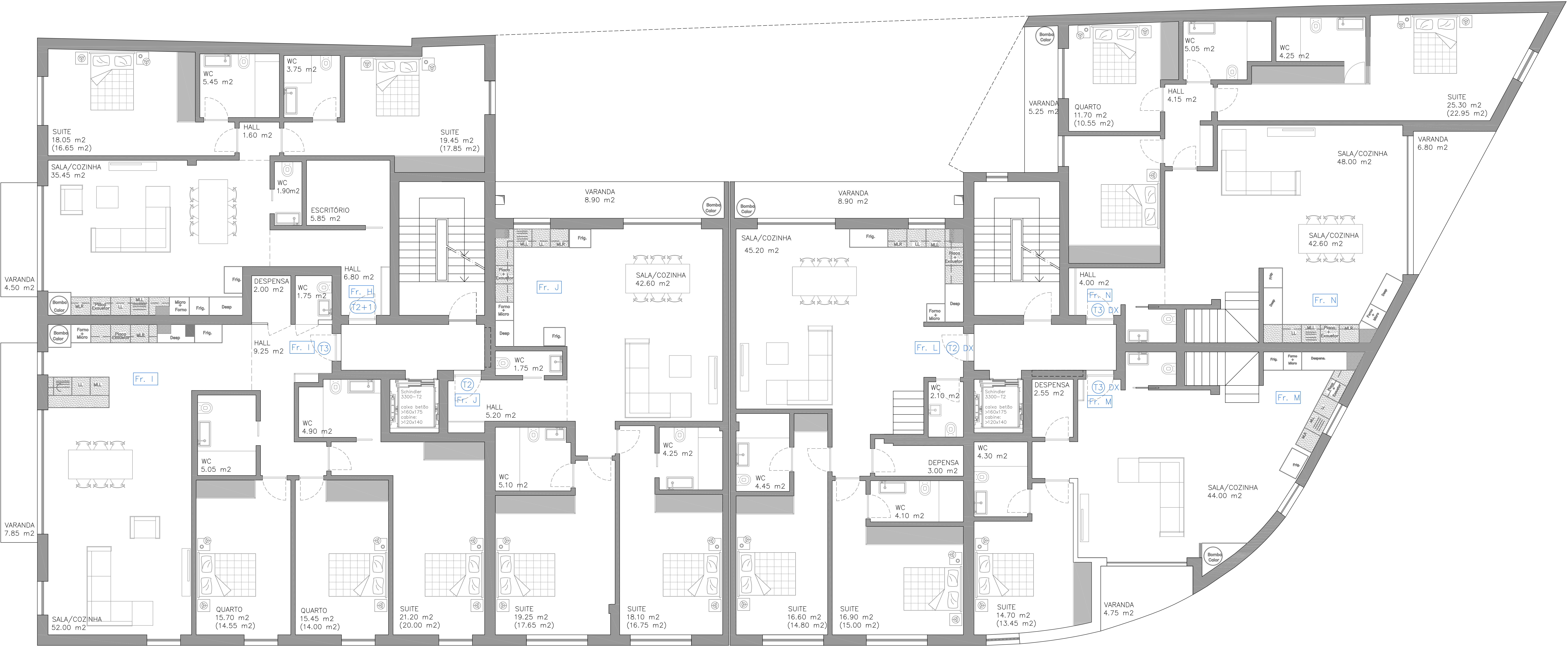
PLANTA DO 1º ANDAR
