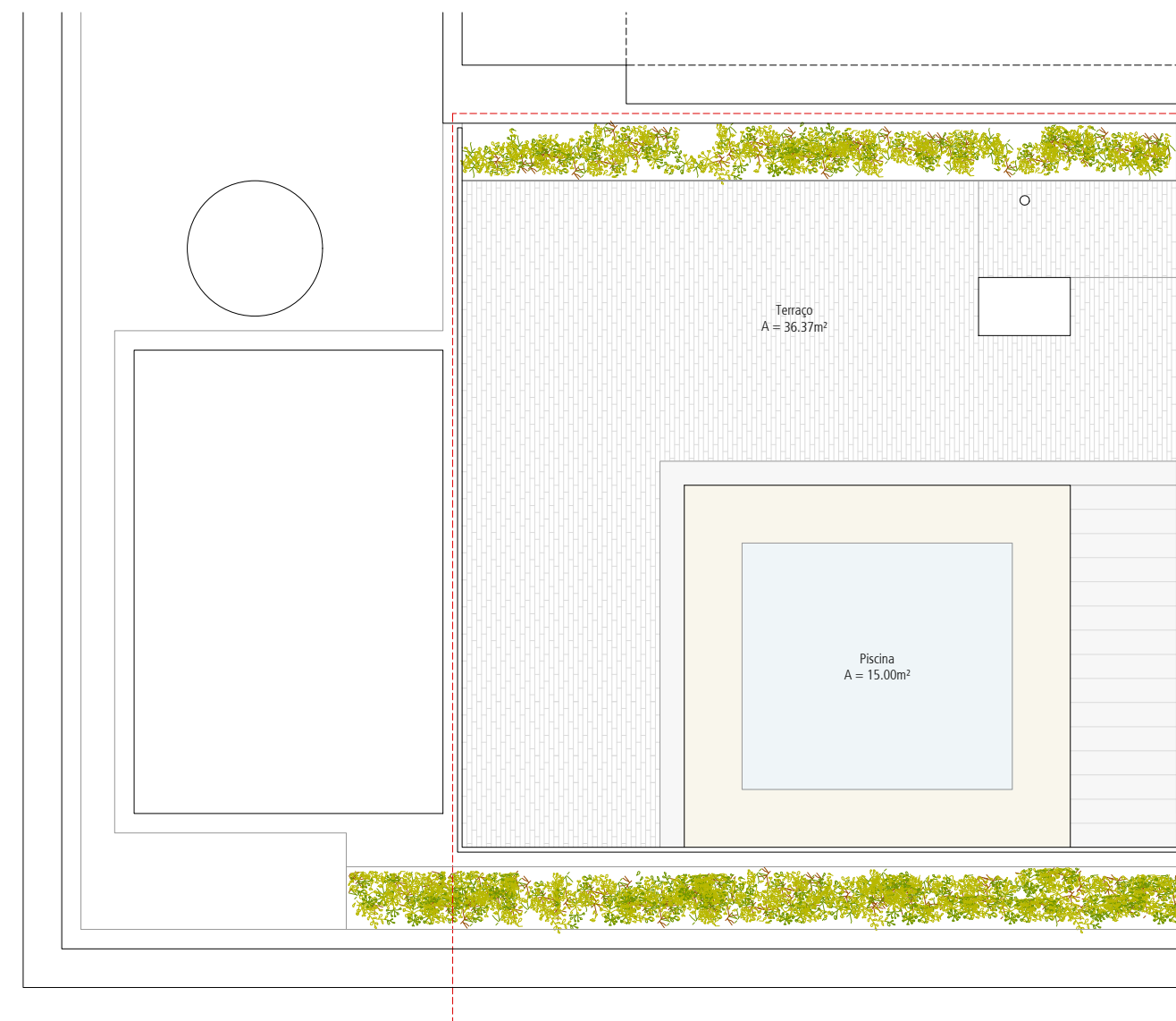
Cobertura . Rooftop
