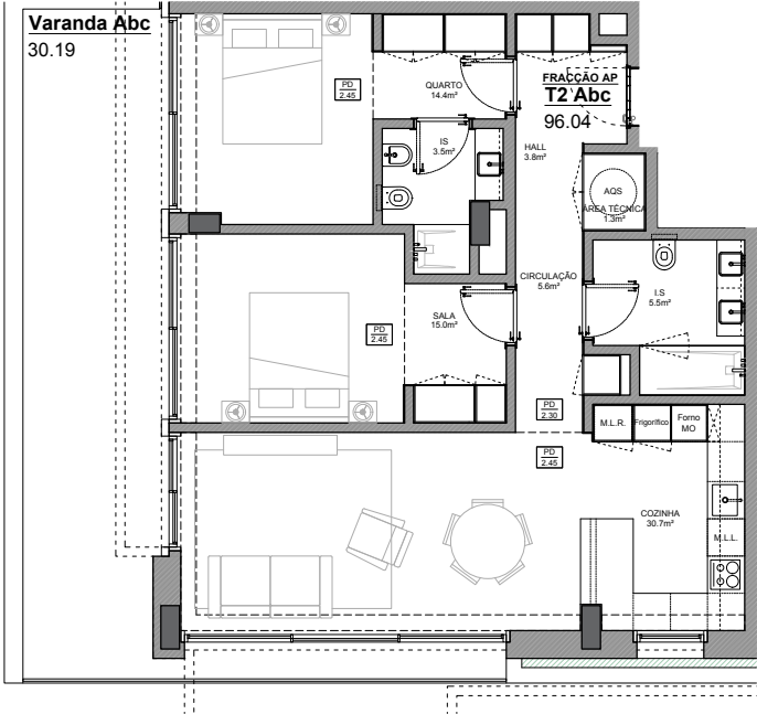
PLANTA 1/100
