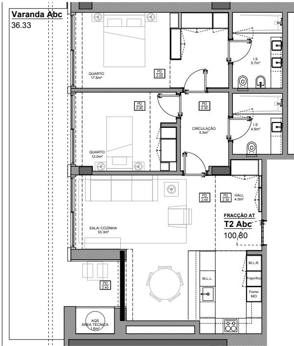
PLANTA 1/100
