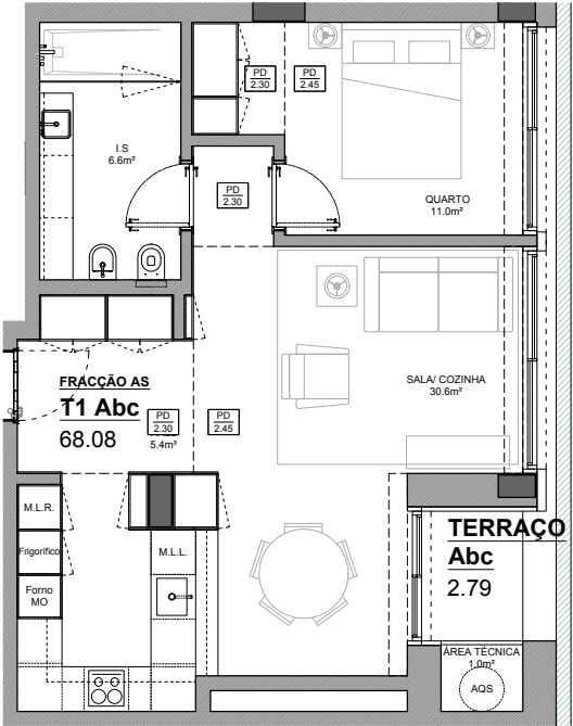
PLANTA 1/100
