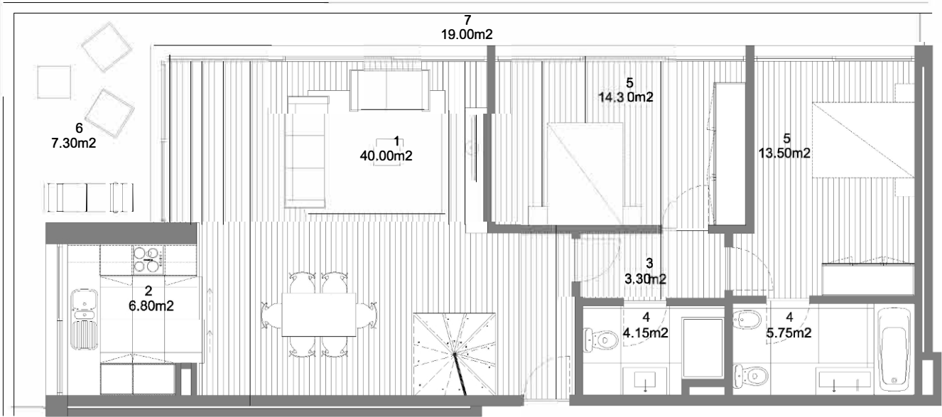
PISO 2 0 1m 2m 3m
