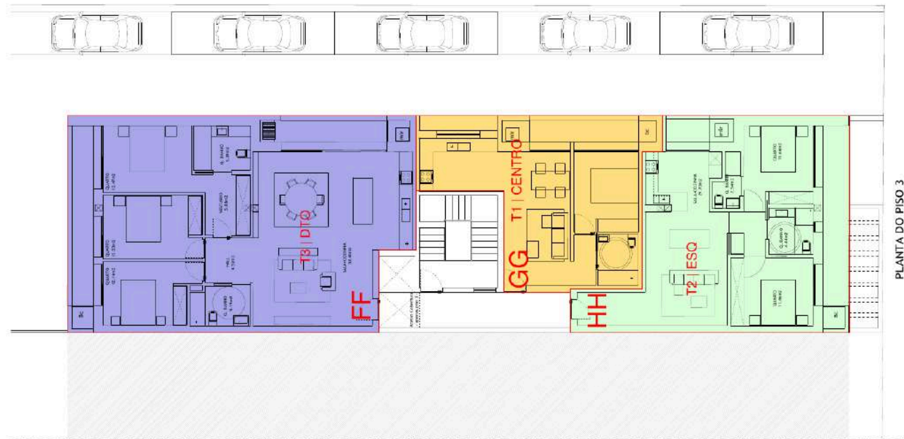
Piso 3
