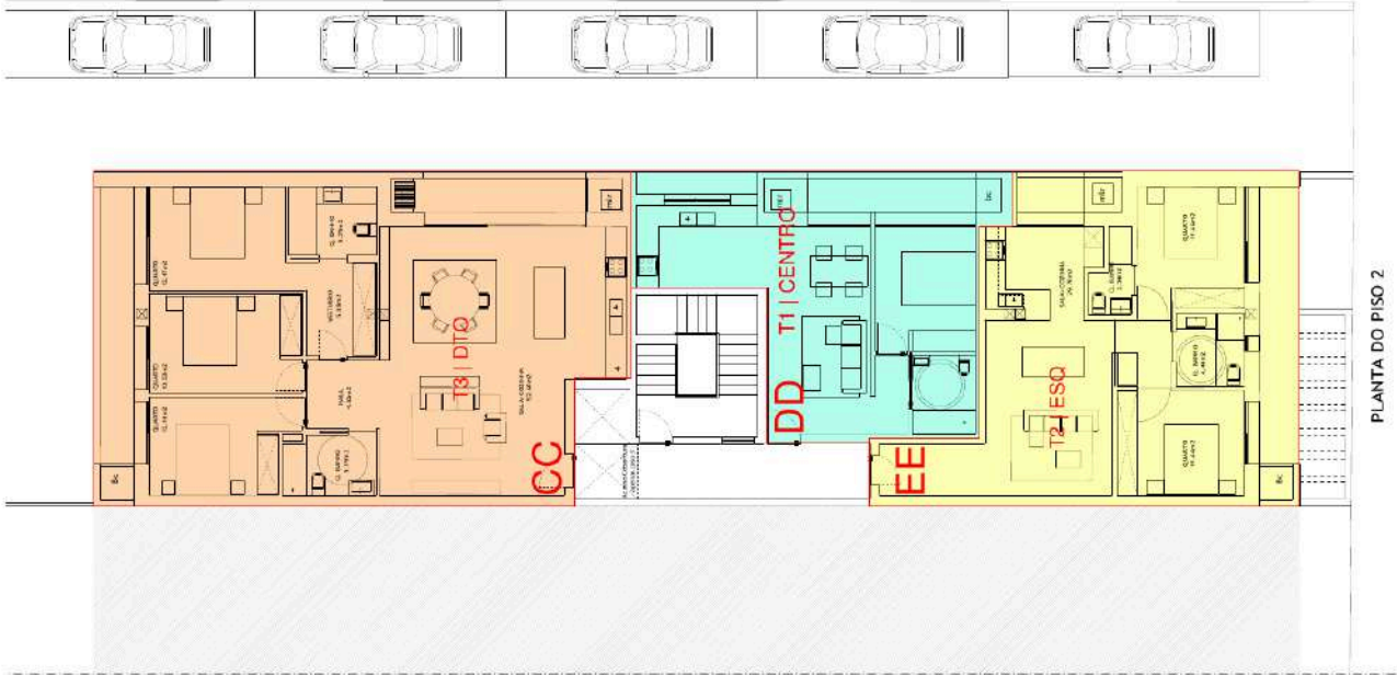
Piso 2
